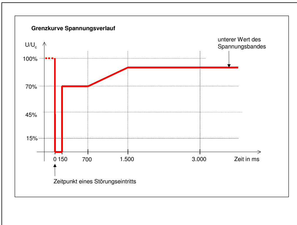
Bild 2.5.1.2-1: Grenzkurve für den Spannungsverlauf am Netzanschlusspunkt für eine Erzeugungsanlage vom Typ 1
